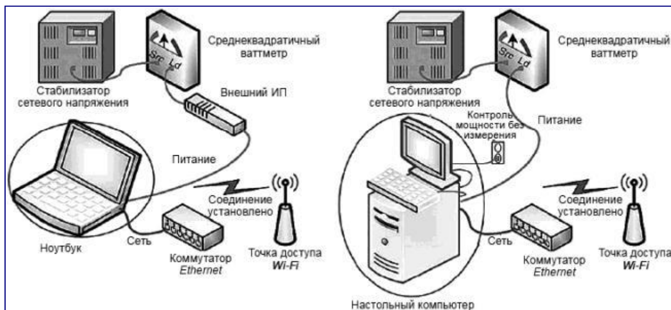
Рисунок 1 - Типичная испытательная установка
