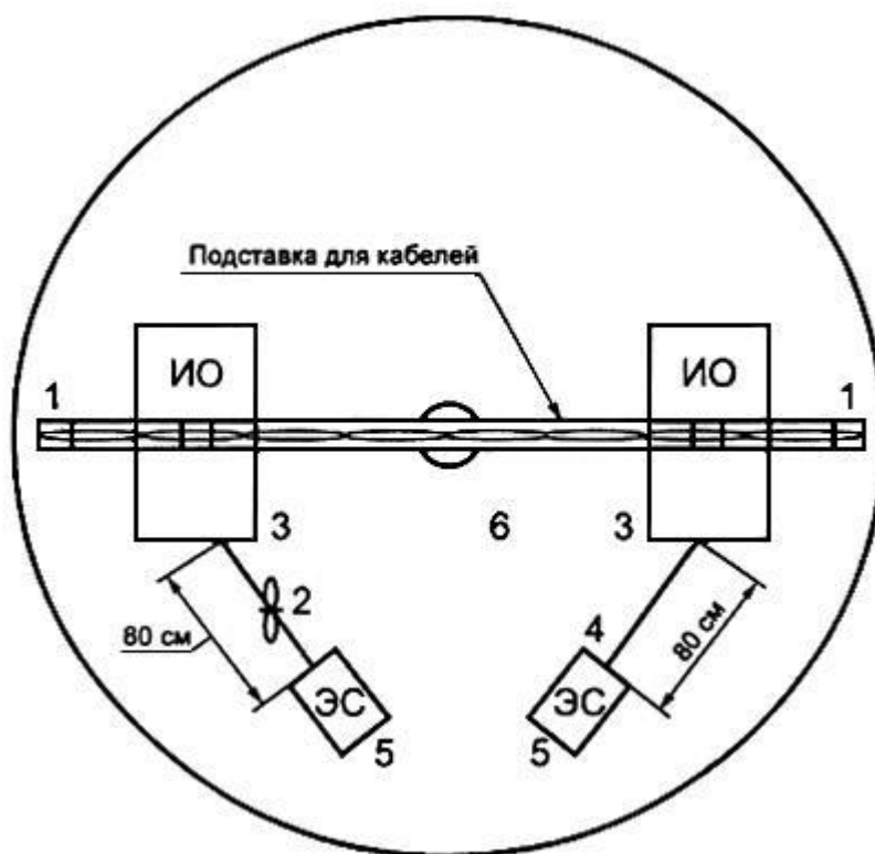
Рисунок 14 - Расположение напольного оборудования с воздушными кабелями при испытаниях (вид сверху)
