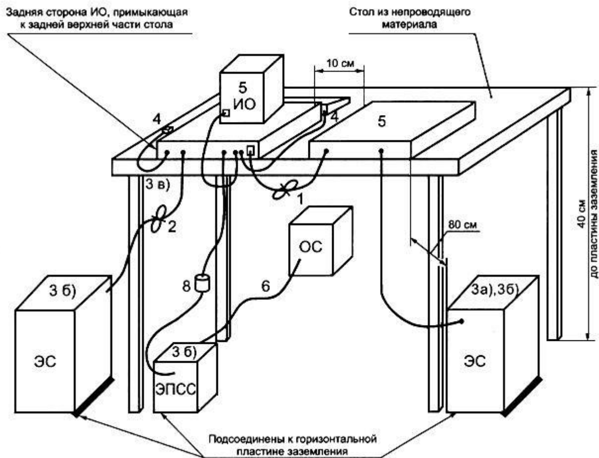
Рисунок 7 - Расположение настольного оборудования при испытаниях (измерение кондуктивных ИРП на измерительной площадке)
