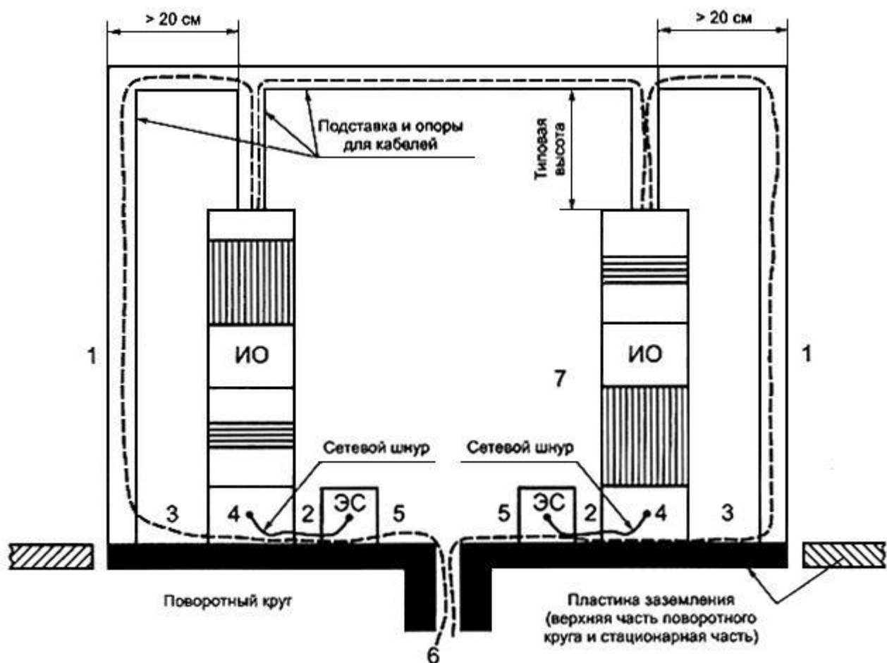
Рисунок 13 - Расположение напольного оборудования с воздушными кабелями при испытаниях (вид сбоку)
