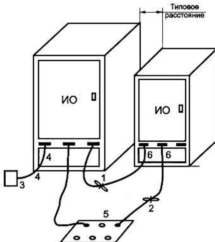
Рисунок 11 - Расположение напольного оборудования при испытаниях (измерение излучаемых ИРП)
