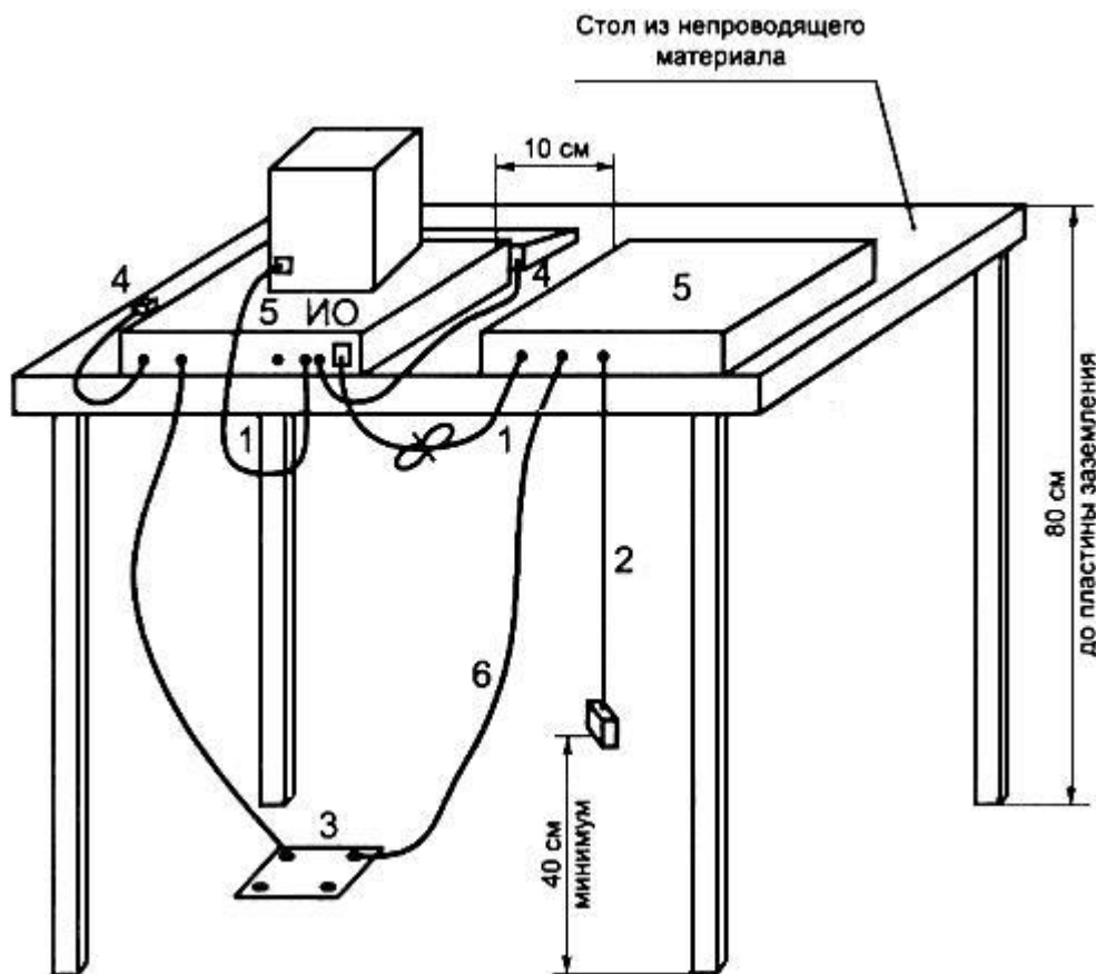
Рисунок 10 - Расположение настольного оборудования при испытаниях (измерение излучаемых ИРП)
