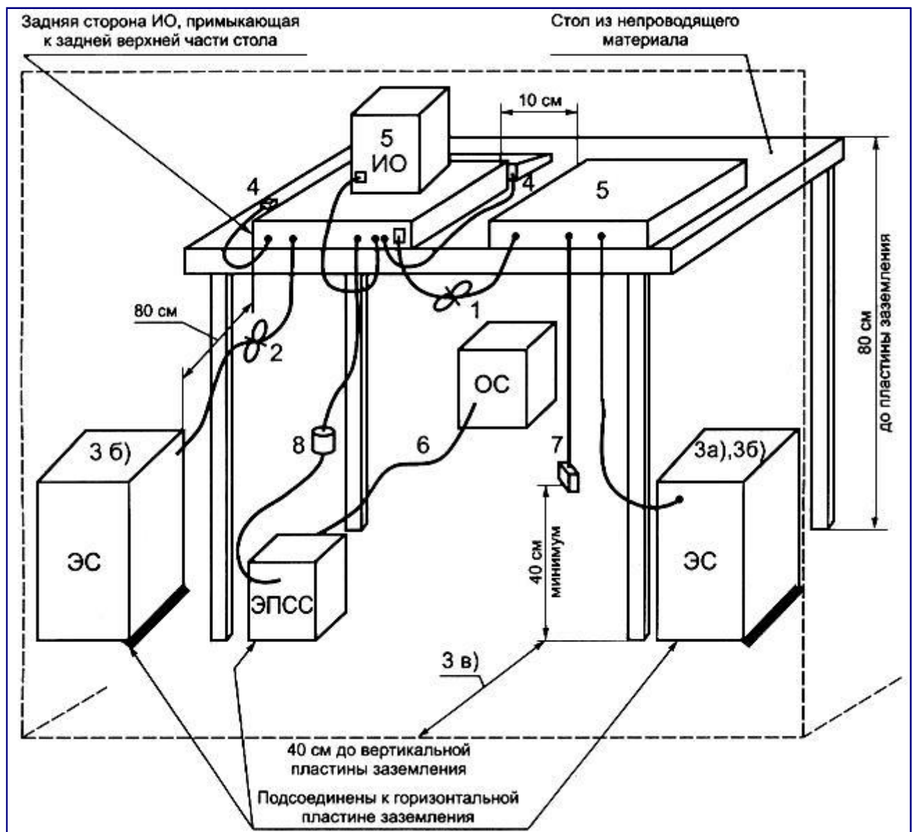
Рисунок 4 - Расположение настольного оборудования при испытаниях (измерение кондуктивных ИРП)
