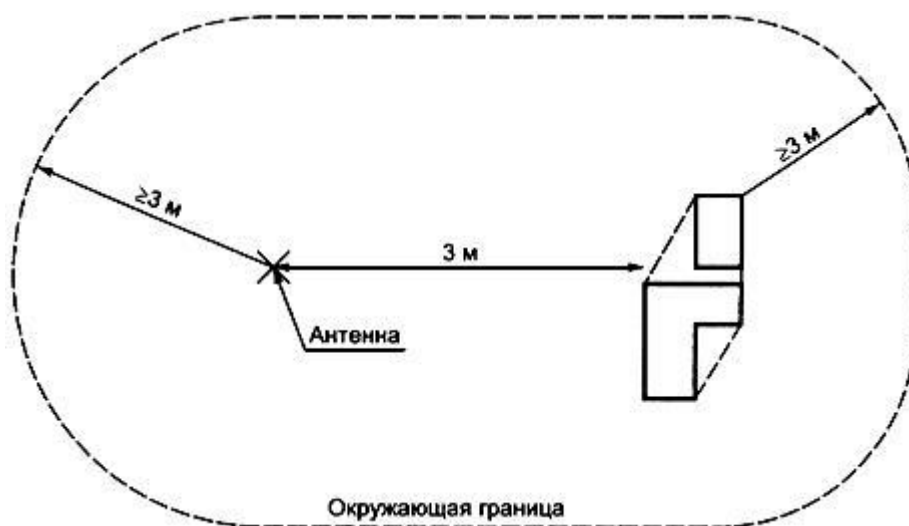
Рисунок 2 - Минимальная альтернативная измерительная площадка
