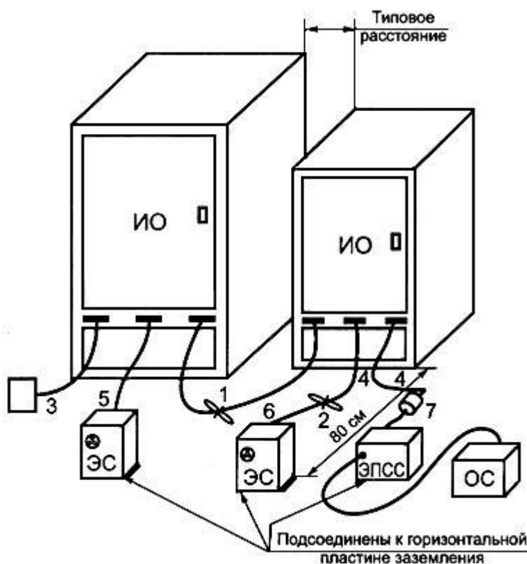
Рисунок 8 - Расположение напольного оборудования при испытаниях (измерение кондуктивных ИРП)
