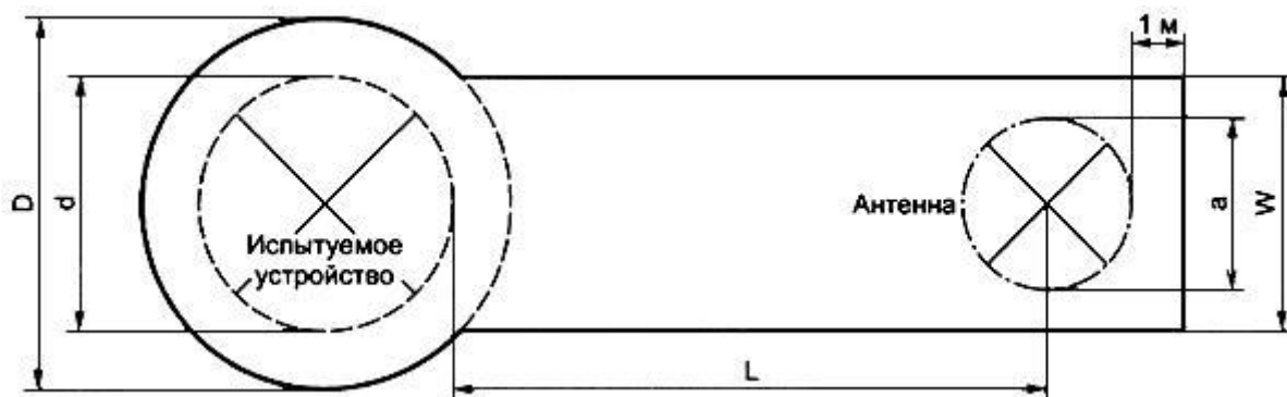
Рисунок 3 - Минимальный размер металлической пластины заземления
