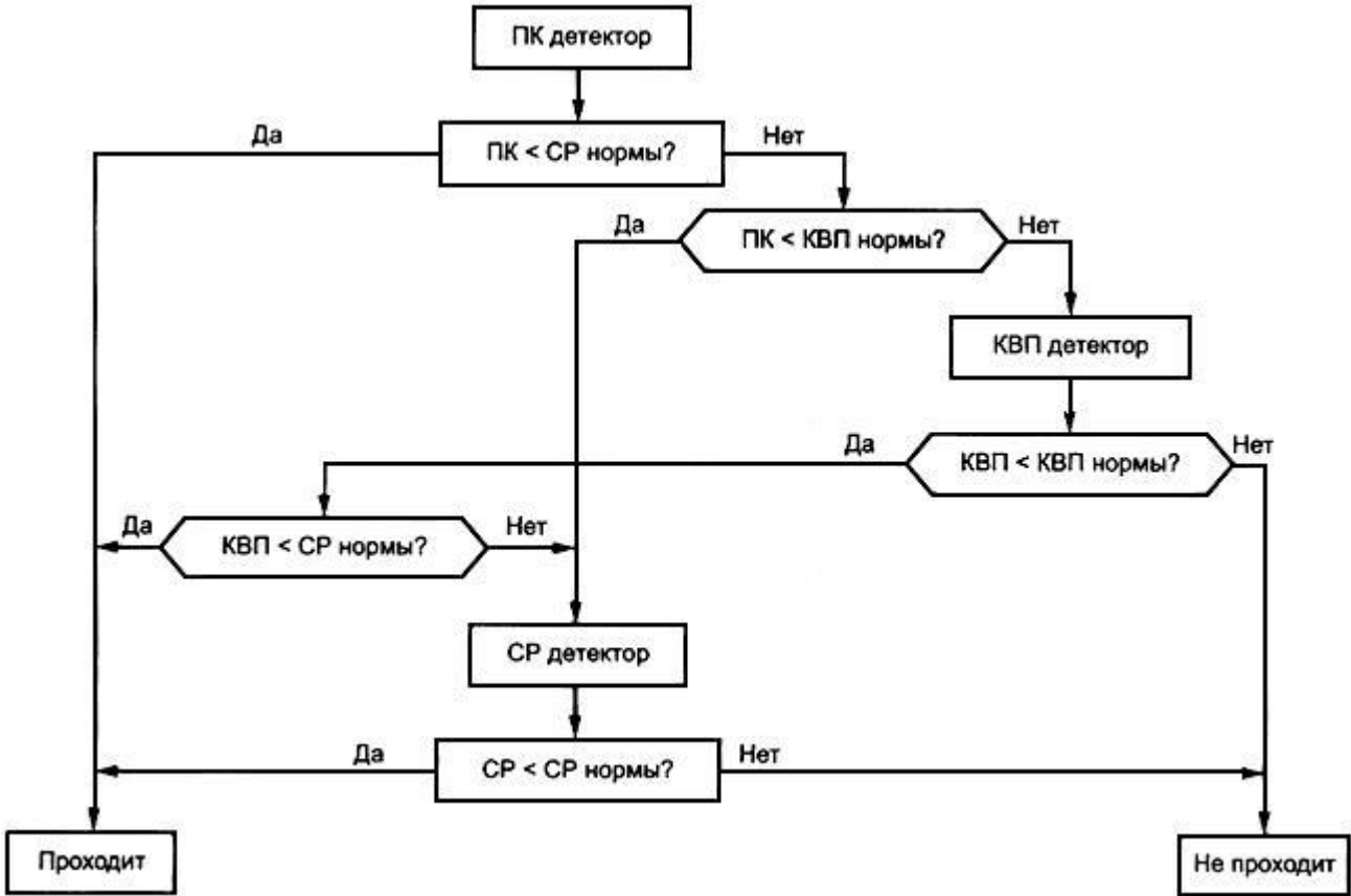
Рисунок А.1 - Алгоритм принятия решения о результатах испытаний ИО при измерениях пиковых значений ИРП
