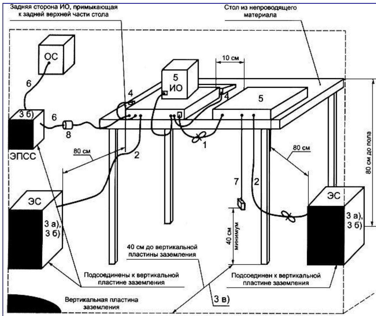
Рисунок 5 - Альтернативное расположение настольного оборудования при испытаниях (измерение кондуктивных ИРП)
