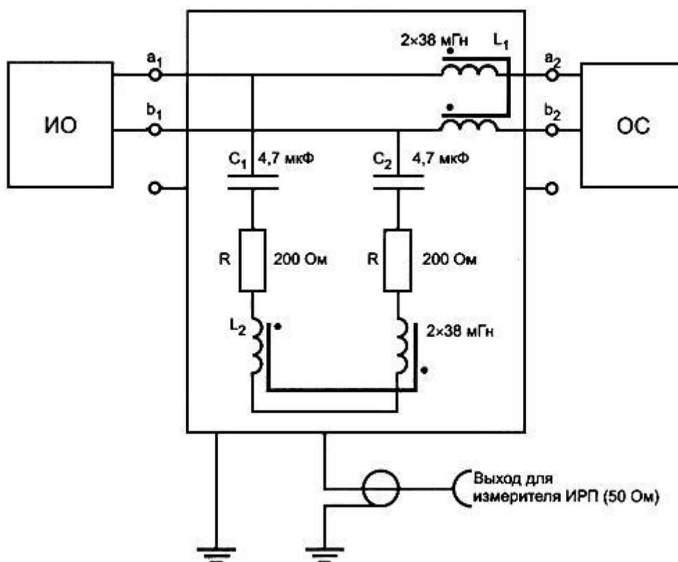
Рисунок В.1 - Эквивалент полного сопротивления сети для применения с одной незранированной симметричной парой
