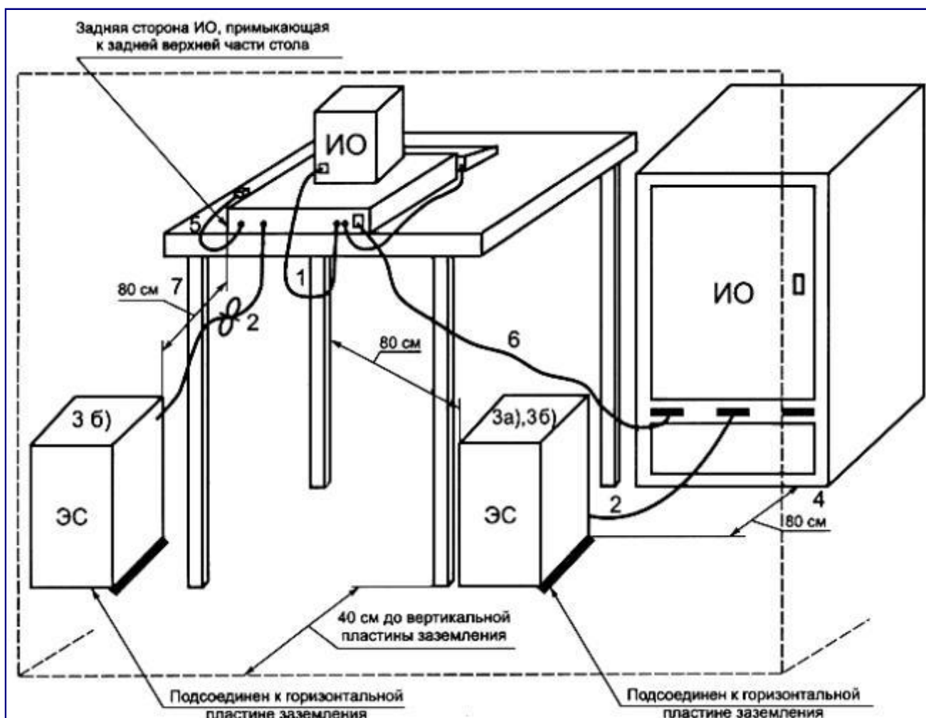
Рисунок 9 - Расположение напольного и настольного оборудования при испытаниях (измерение кондуктивных ИРП)
