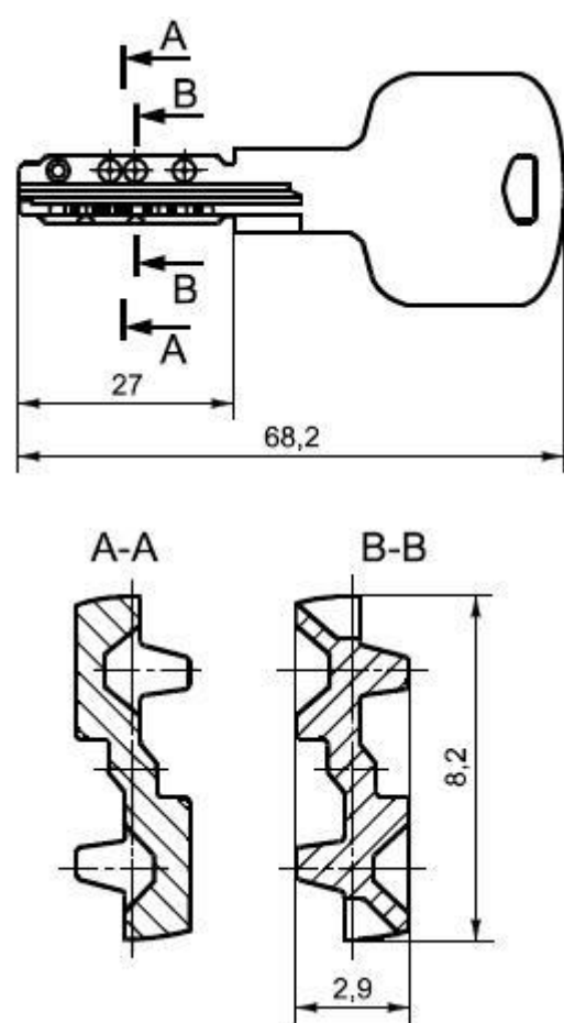
Рисунок Б.25 - Пример ключа цилиндрического механизма
