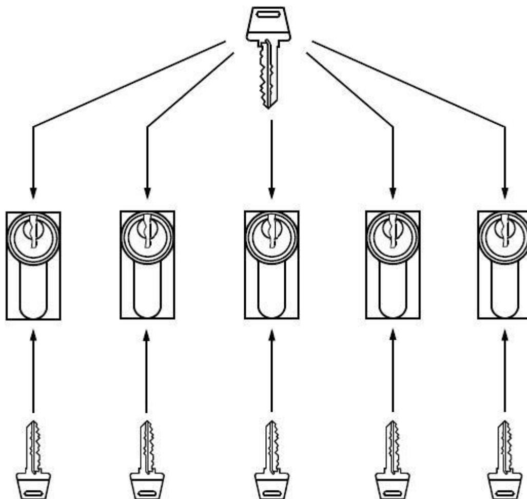
Рисунок А.3 - Система цилиндровых механизмов с групповым ключом
