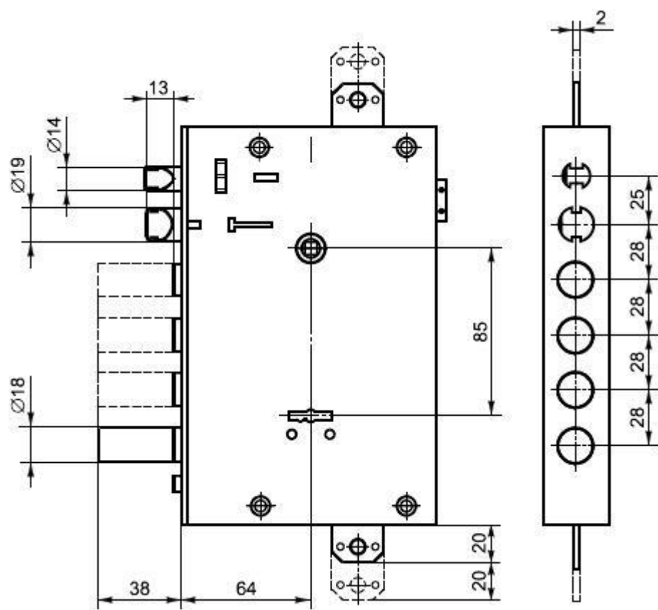
Рисунок Б.10 - Пример сувальдного врезного электромеханического замка
