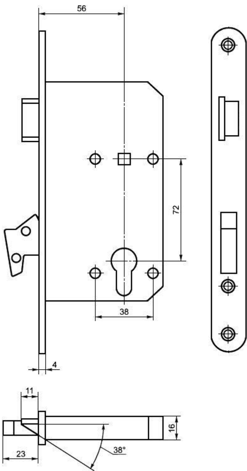
Рисунок Б.3 - Пример цилиндрического врезного замка типа ЗВ4 с крюкообразным засовом
