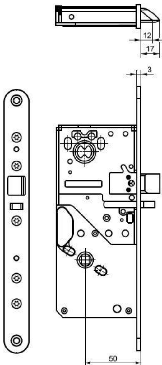
Рисунок Б.11 - Пример электромеханического моторного врезного замка типа ЗЭМв
