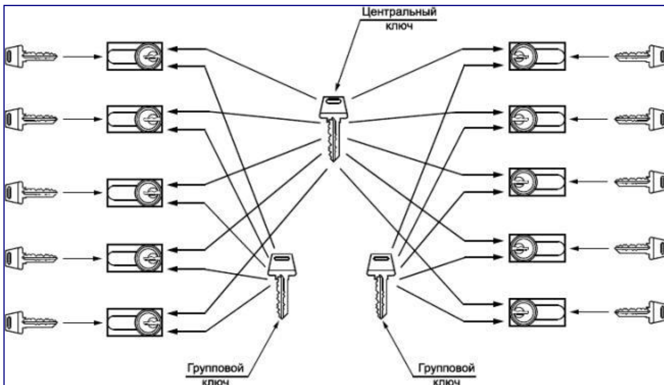
Рисунок А.4 - Система цилиндрических механизмов с центральным ключом
