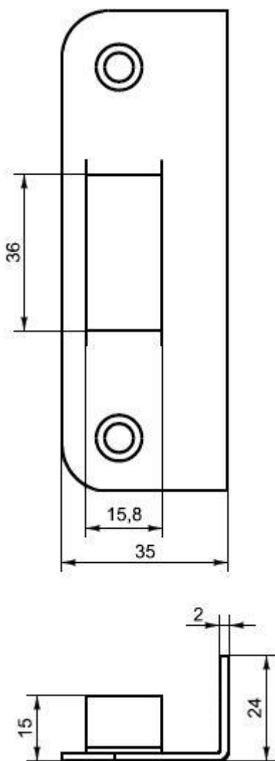
Рисунок Б.16 - Пример запорной угловой планки
