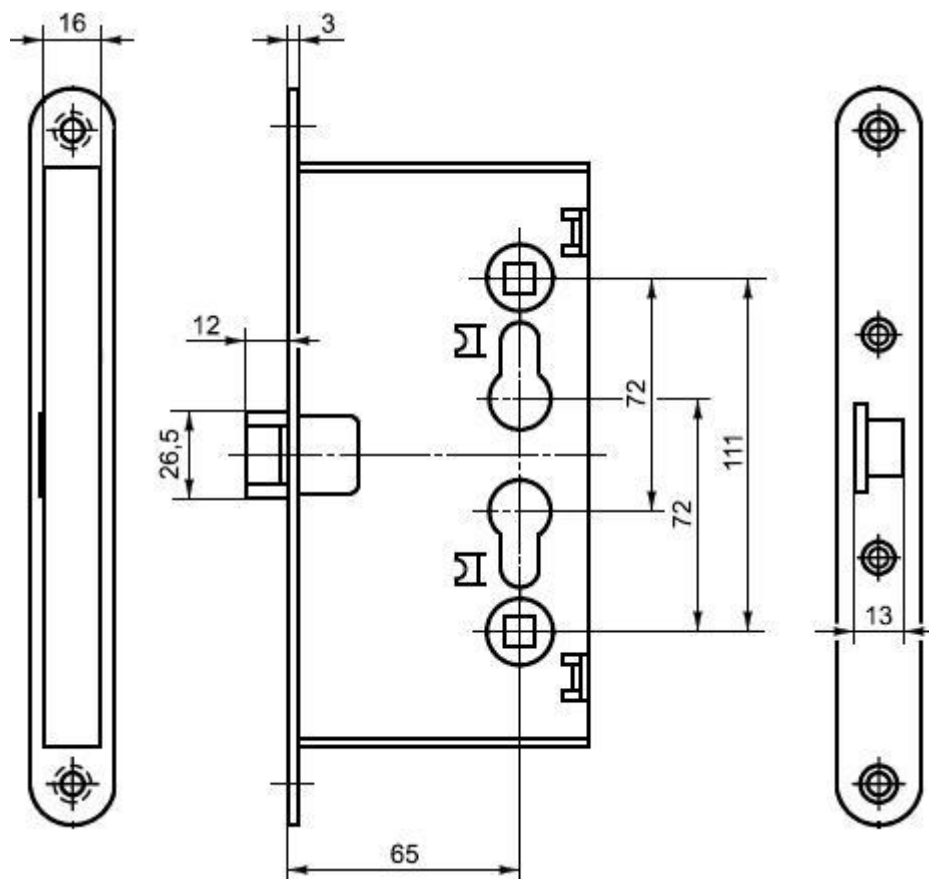
Рисунок Б.12 - Пример замка для противопожарной двери
