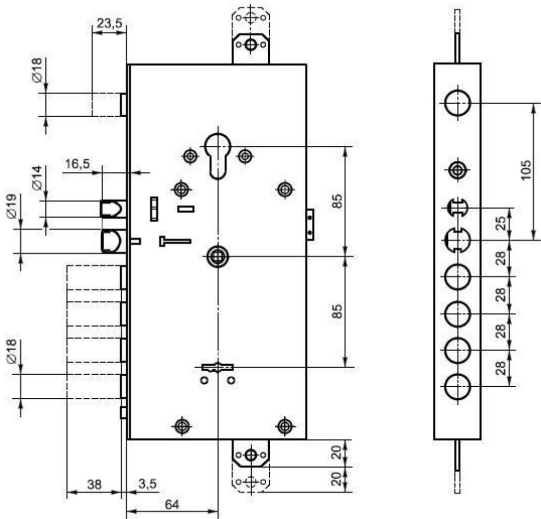
Рисунок Б.7 - Пример комбинированного врезного электромеханического замка
