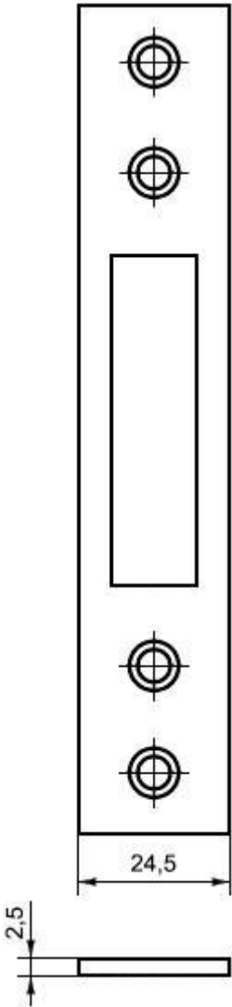
Рисунок Б.14 - Пример простой запорной планки
