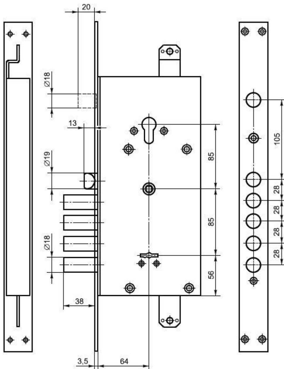
Рисунок Б.8 - Пример комбинированного врезного замка типа ЗВ13 с цилиндрическим и сувальдным механизмами
