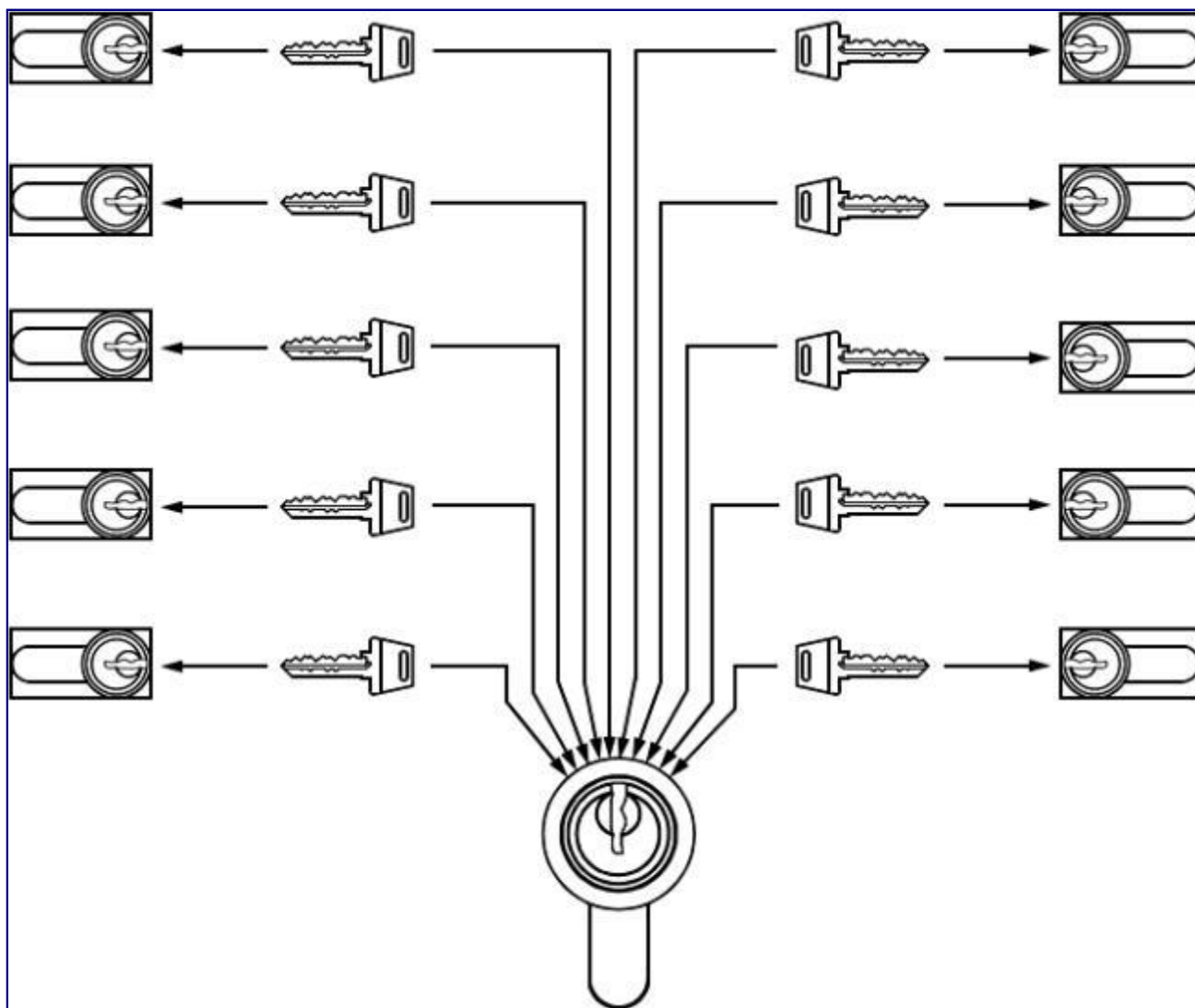
Рисунок А.5 - Система цилиндрических механизмов с центральным механизмом
