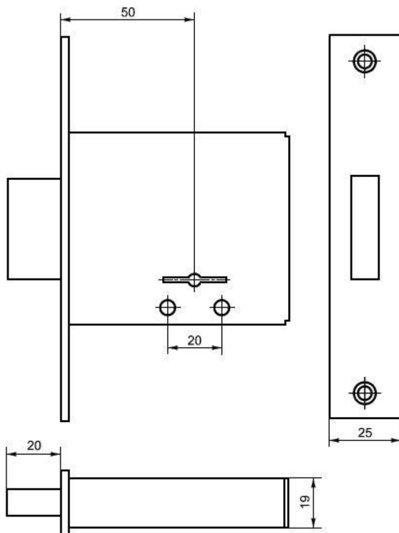
Рисунок Б.5 - Пример сувальдного врезного замка типа ЗВ8
