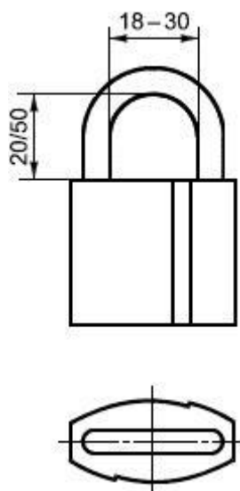
Рисунок Б.13 - Пример навесного замка типа ЗНВ1
