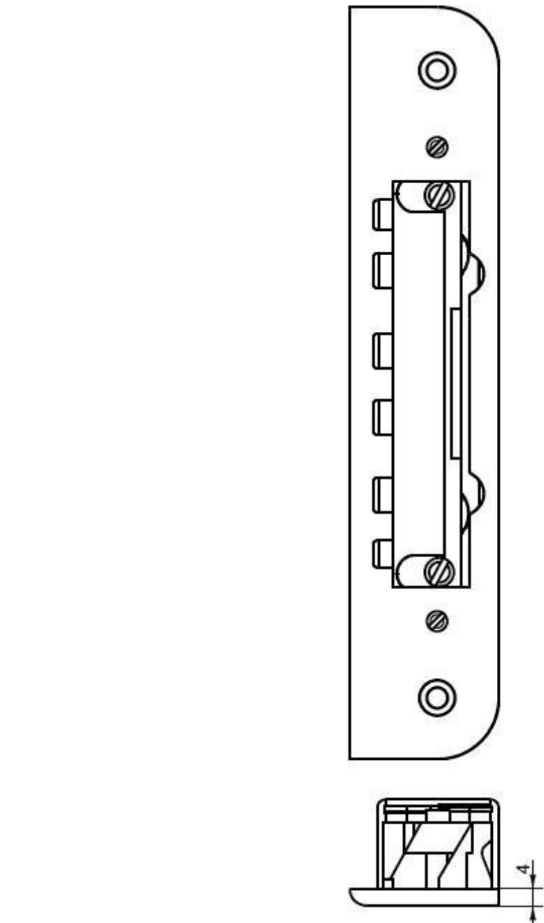
Рисунок Б.17- Пример усиленной запорной планки коробчатой формы
