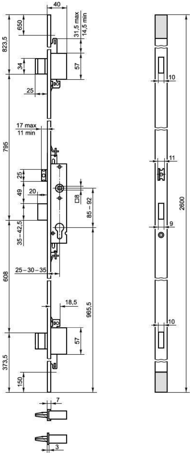
Рисунок Б.22 - Пример многозапорного замка
