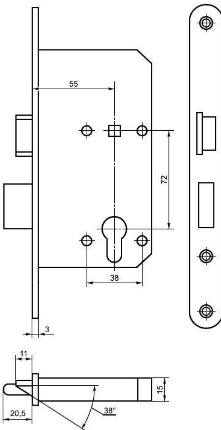
Рисунок Б.4 - Пример цилиндрического врезного замка типа ЗВ7
