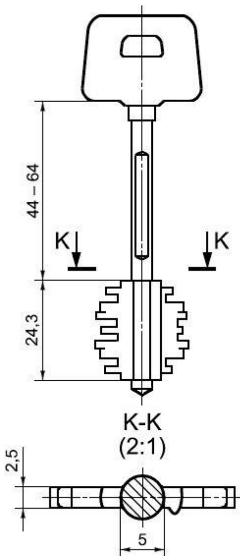
Рисунок Б.20 - Пример ключа сувальдного замка
