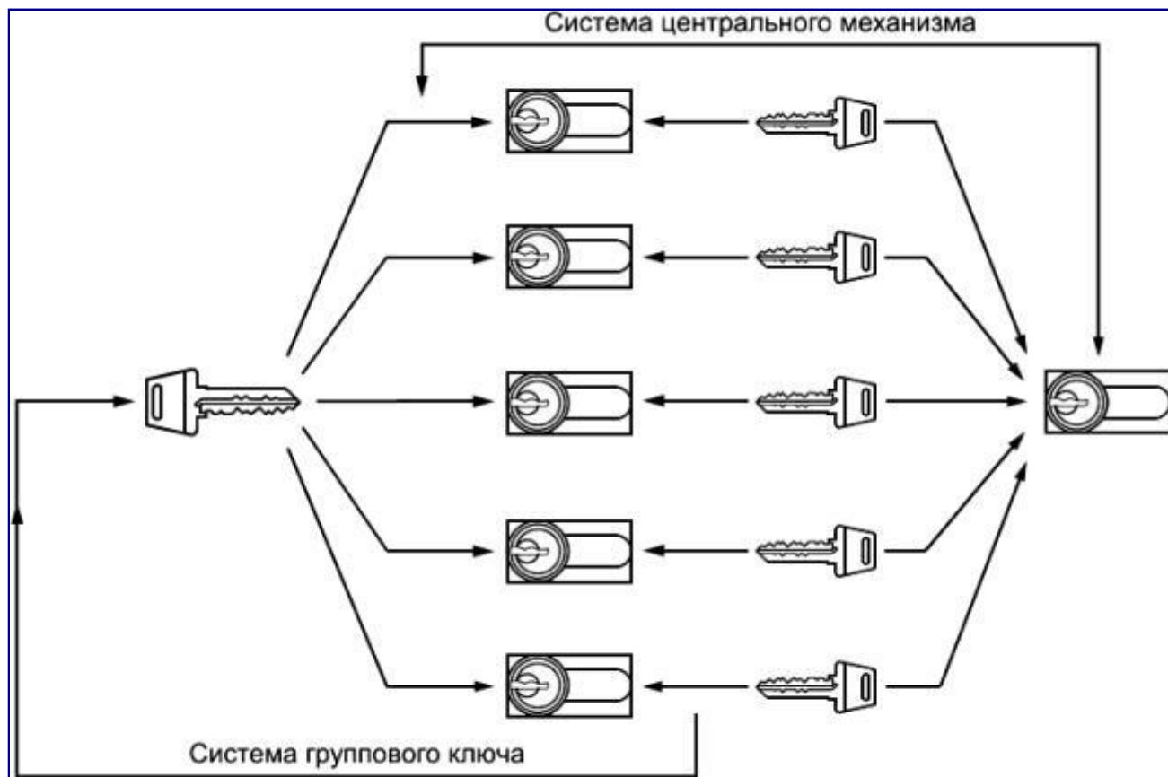
Рисунок А.6 - Смешанная система цилиндрических механизмов
