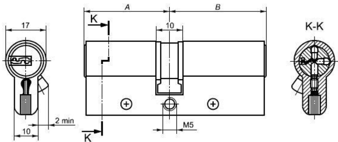
Рисунок Б.21 - Пример двухстороннего цилиндрического механизма
