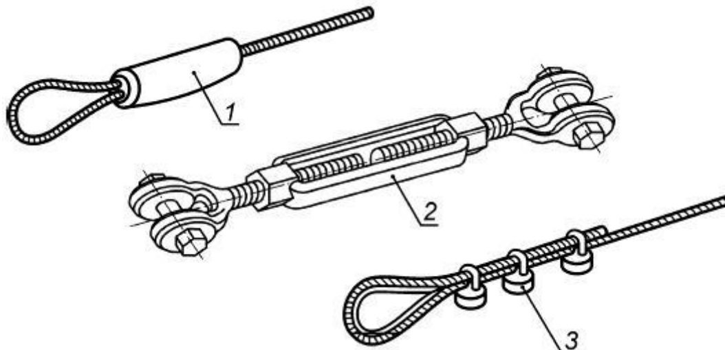
Рисунок 18 - Опрессованная петля, талреп, петля с коушем и зажимами
