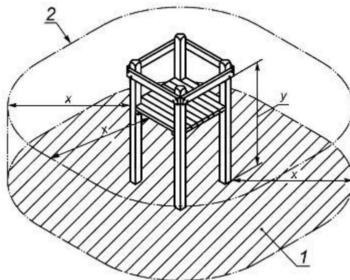
Рисунок 16 - Зоны падения платформы и шеста
