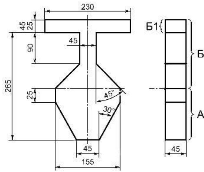
Рисунок Г.3 - Шаблон для определения застревания головы или шеи ребенка в прямоугольных и V-образных зазорах
