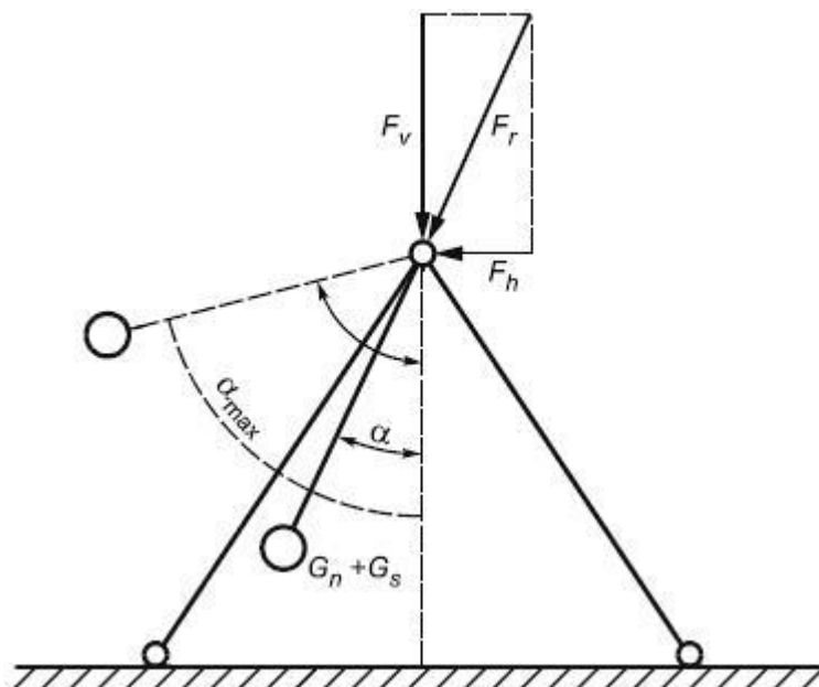
Рисунок А.2 - Силы, действующие на качели
