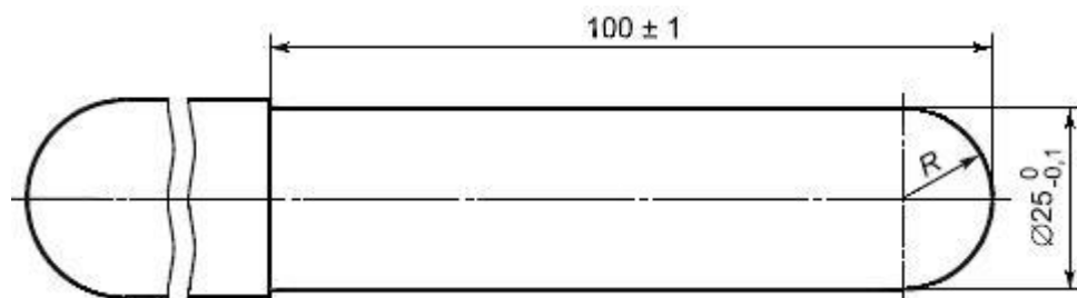
Рисунок Г.13 - Стержень-палец Б (большой)
