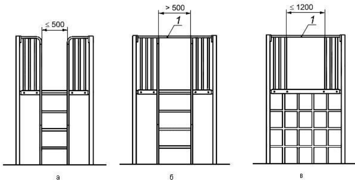
Рисунок 8 - Проемы в ограждениях
