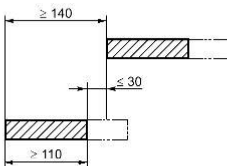
Рисунок 17 - Проекция и глубина ступени
