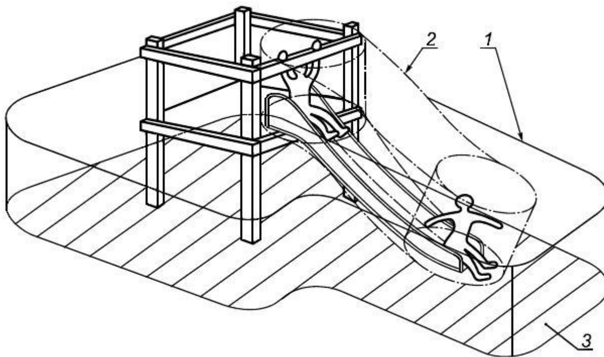
Рисунок 1 - Зоны игрового оборудования
