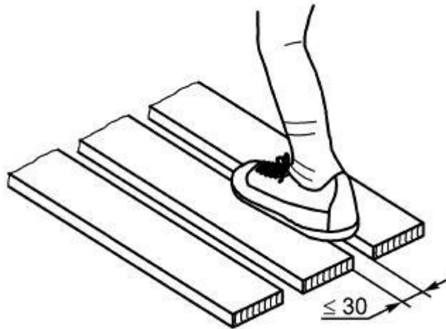
Рисунок 10 - Ширина зазоров на поверхностях наклоном до 45°
