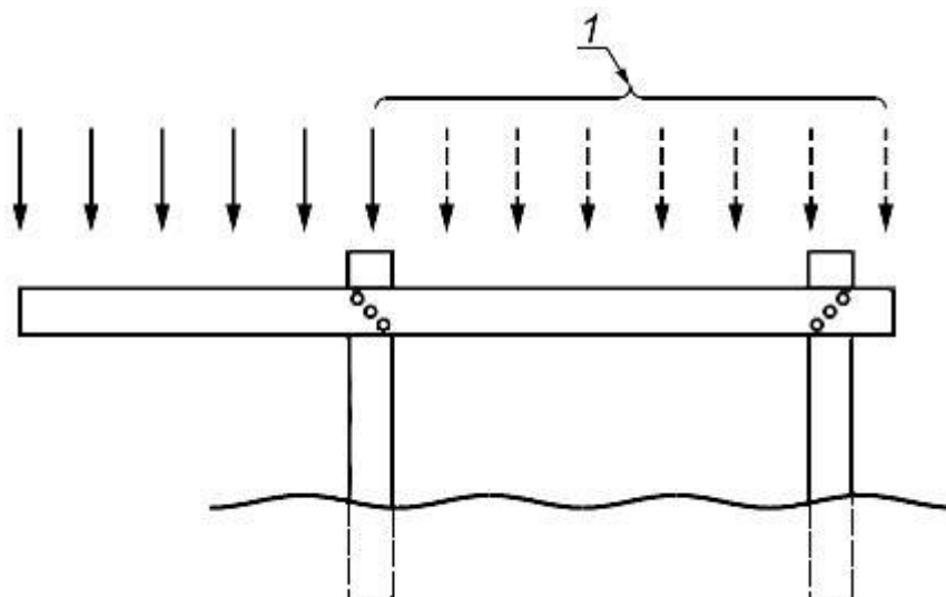
Рисунок 5 - Удаление части нагрузки
