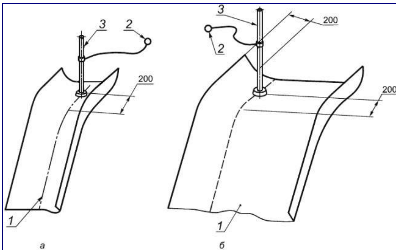
Рисунок Г.10 - Размещение испытательного устройства на горке
