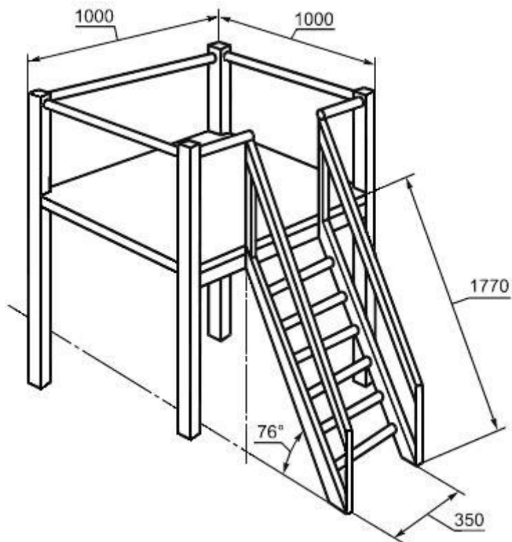
Рисунок А.1 - Платформа с лестницей
