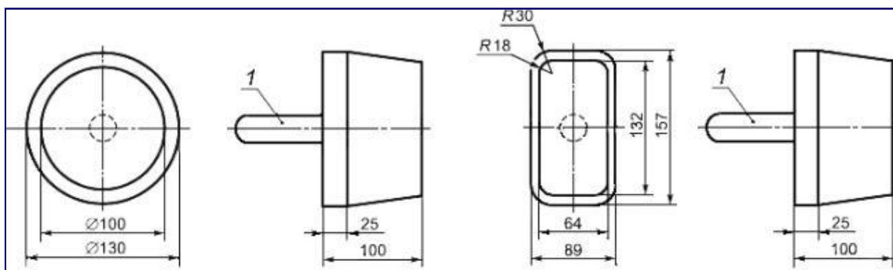
Рисунок Г.1 - Малые щупы для определения застревания головы или шеи ребенка в отверстиях
