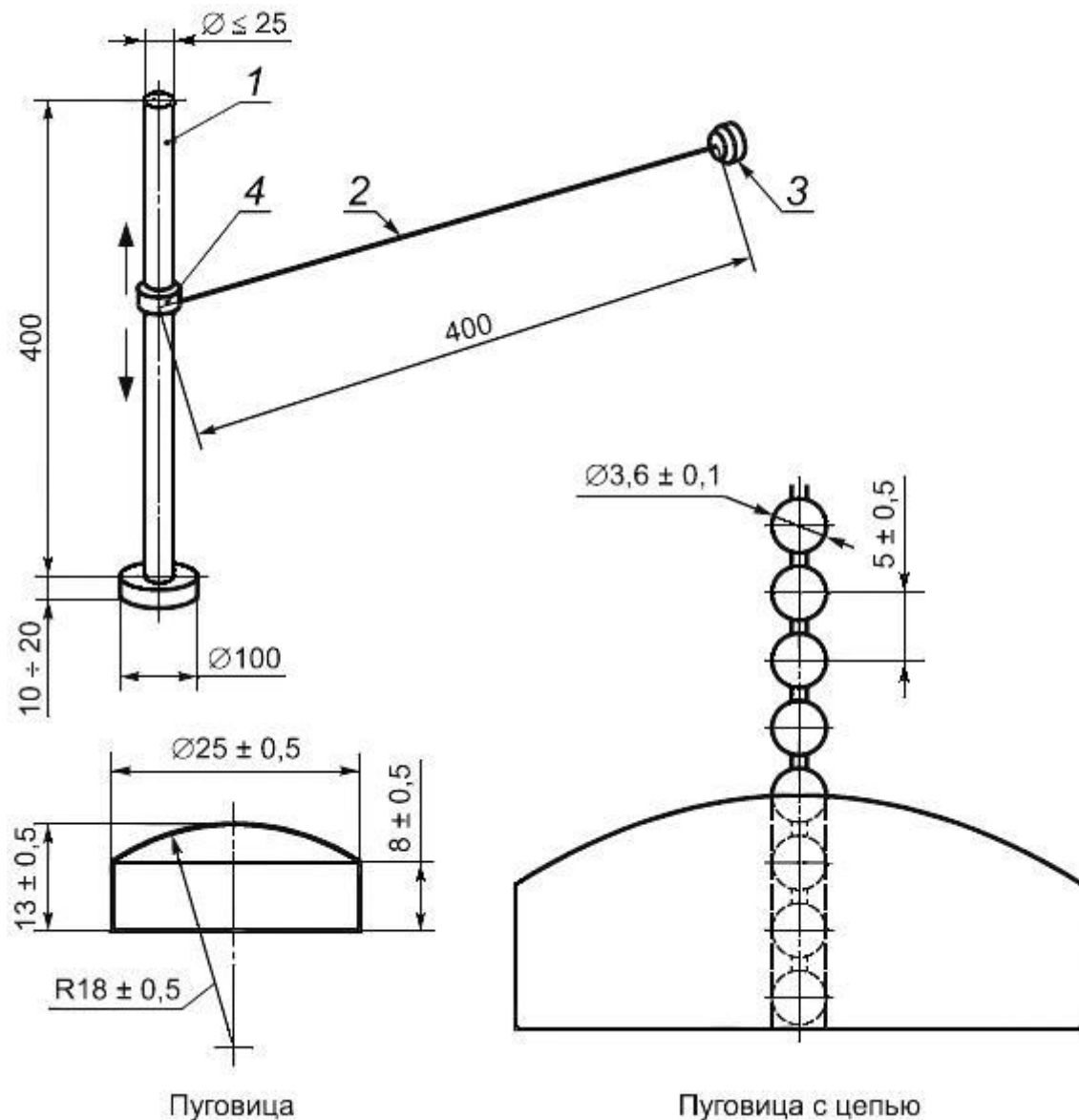
Рисунок Г.9 - Испытательное устройство для испытаний застревания пуговицы
