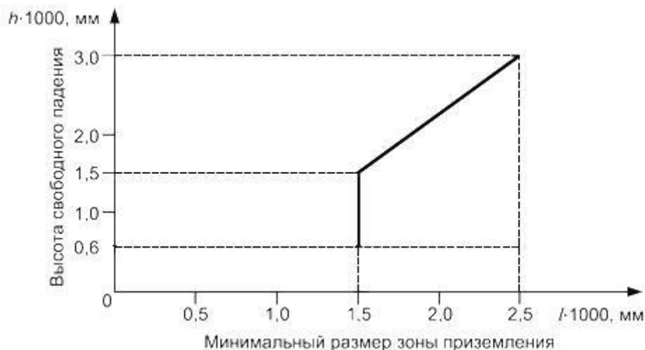
Рисунок 14 - Размеры зоны приземления
