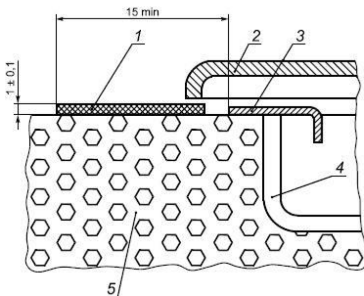
Рисунок 19 - Устройство для испытания крышек и закрывающих пластин
