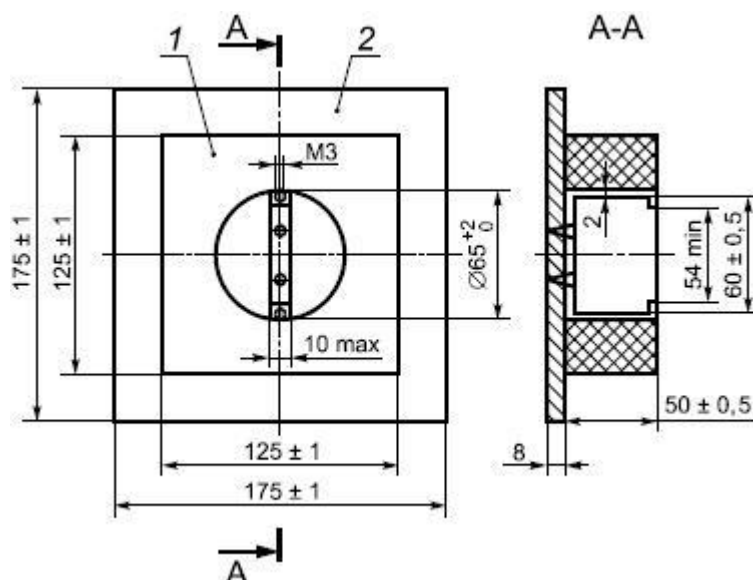
Рисунок 18 - Основание для крепления выключателей скрытой установки
