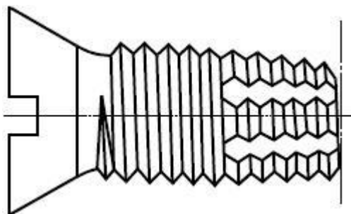
Рисунок 7 - Самонарезающий режущий винт
