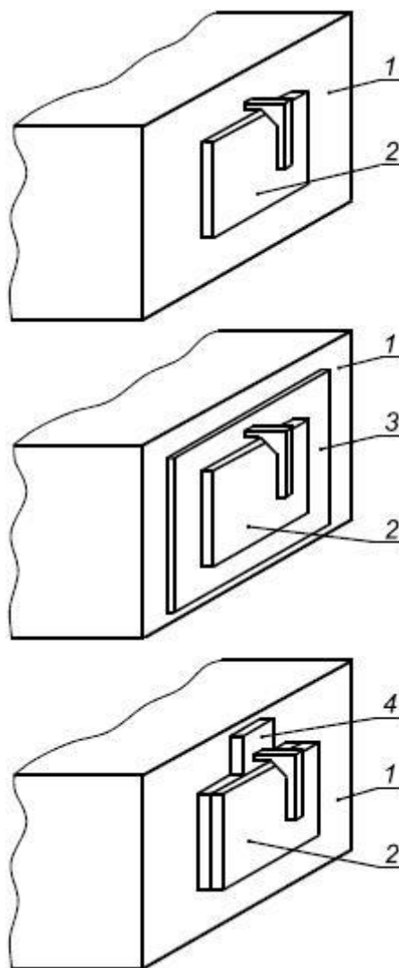
Рисунок 21 - Пример использования калибра на рисунке 20, установленного за выключателем, который смонтирован на монтажной или опорной поверхности
