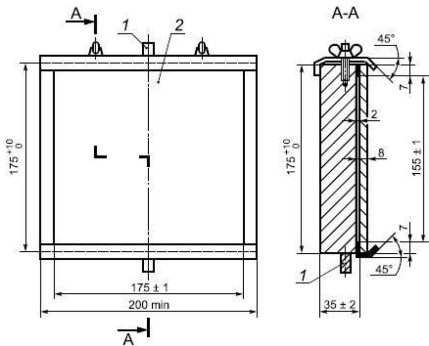
Рисунок 17 - Основание для крепления образца
