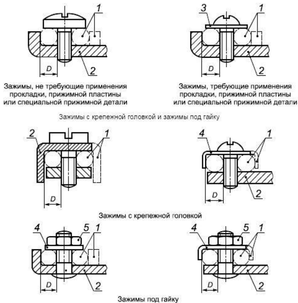
Рисунок 2 - Зажимы с крепежной головкой и зажимы под гайку
