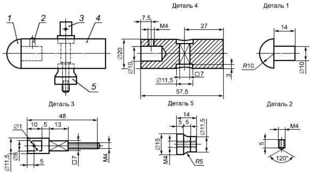
Рисунок 16 - Устройство маятника для испытания на удар
