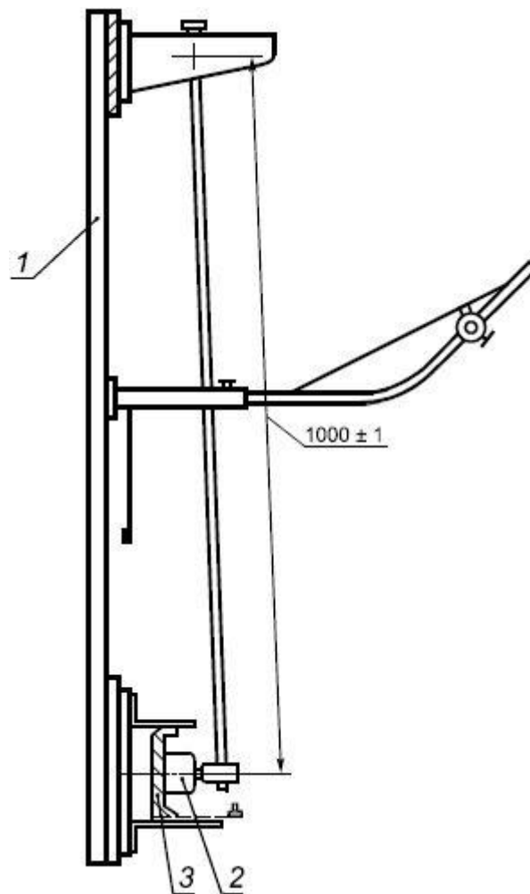
Рисунок 15 - Устройство для испытания на удар
