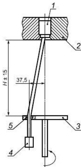
Рисунок 10 - Испытательное устройство для контроля повреждения проводников
