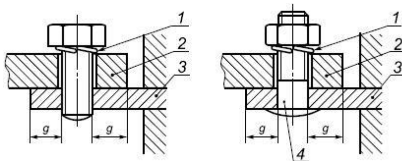
Рисунок 4 - Зажимы под наконечник
