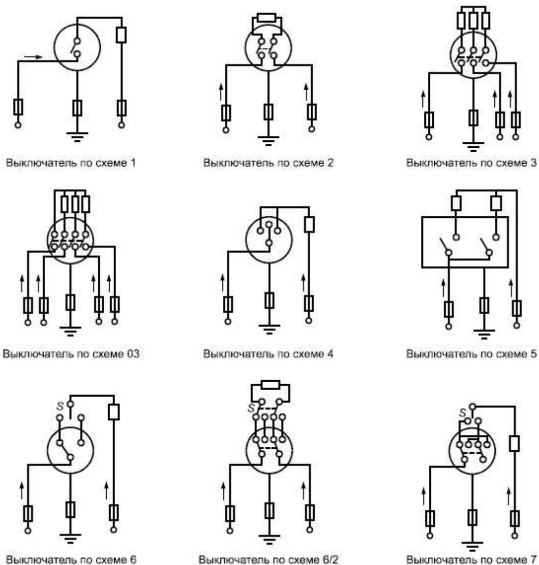
Рисунок 13 - Электрические схемы для проверки выключающей и разрывной мощности и нормальной работы выключателя
