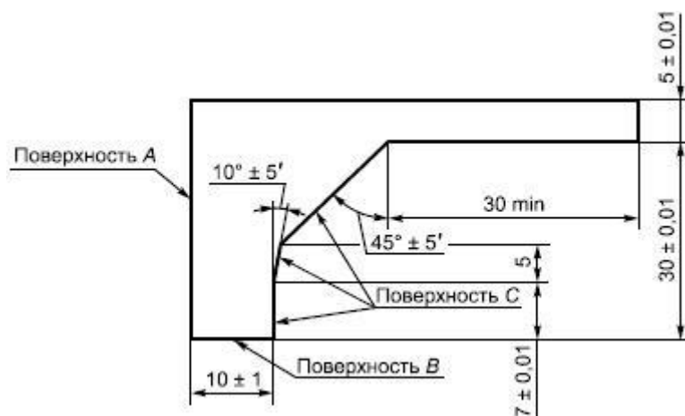
Рисунок 20 - Калибр (толщина около 2 мм) для проверки габаритов крышек для закрывающих пластин
