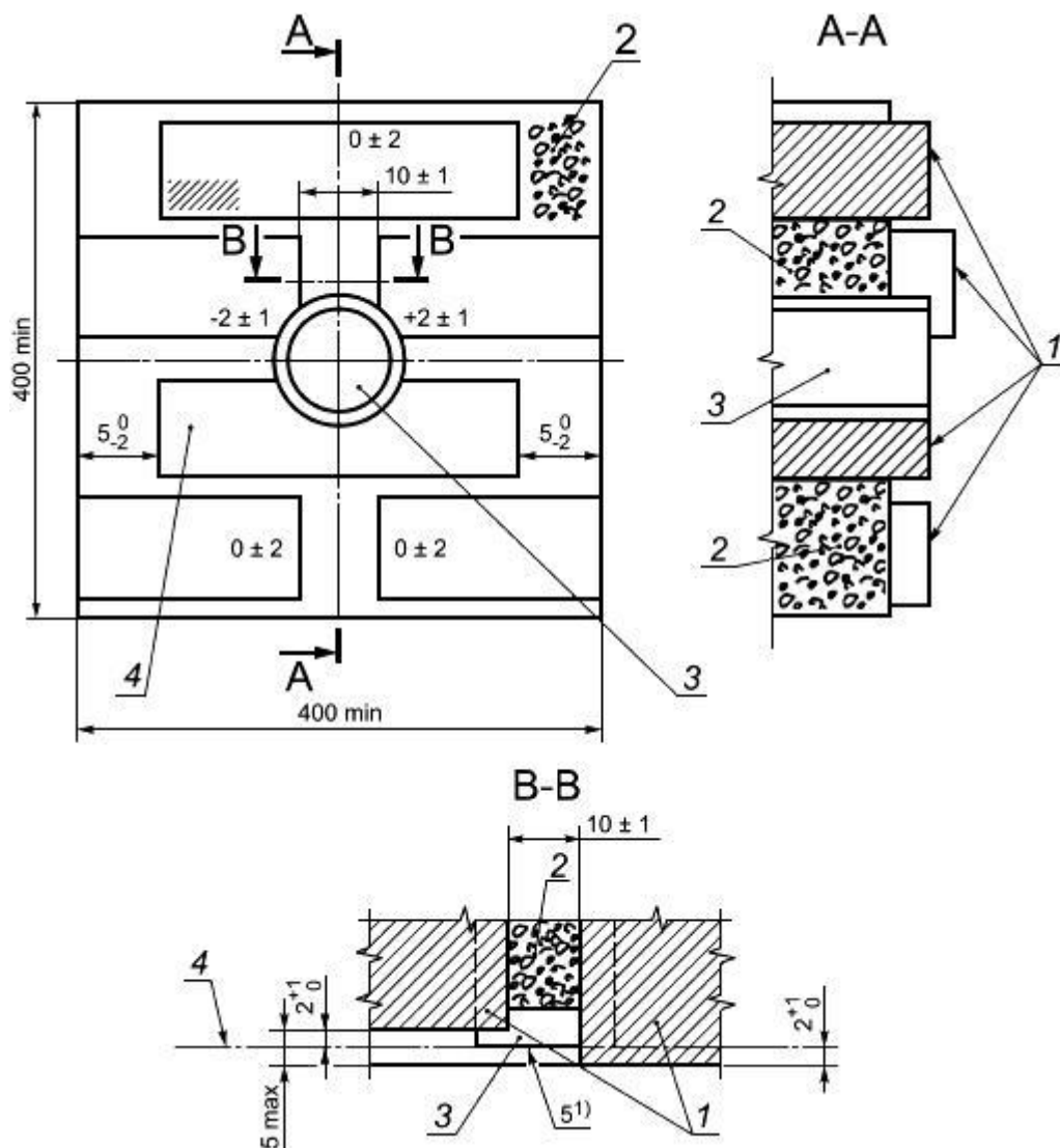
Рисунок 27 - Блок испытательной стены для проведения испытаний в соответствии с требованиями 15.2.2
